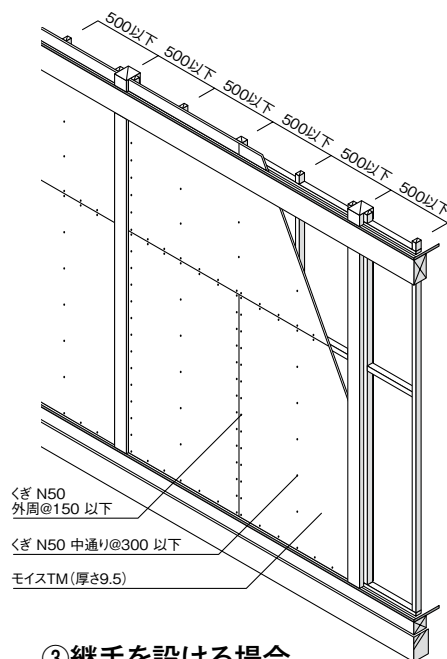
③継手を設ける場合 (上部横張り)
