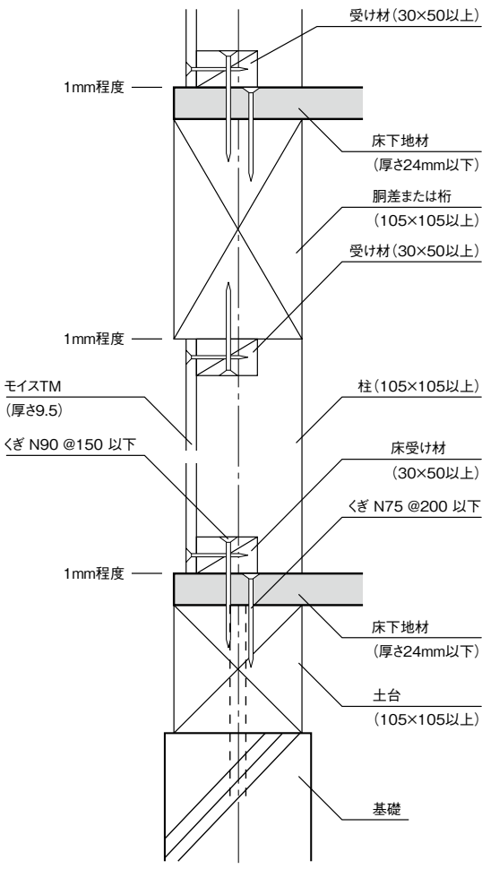
垂直断面図
