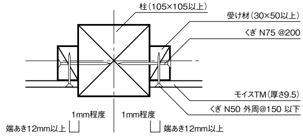
A部詳細図
