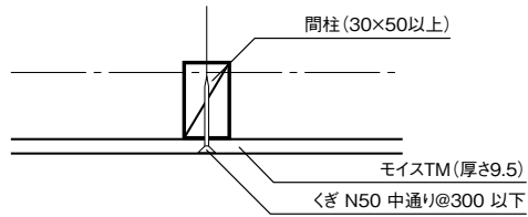
C部詳細図
