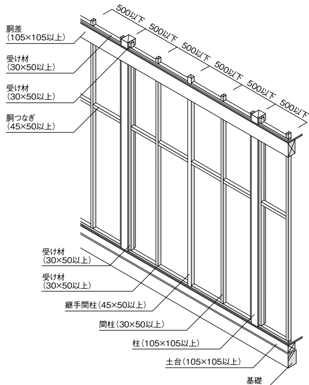
下地組図
